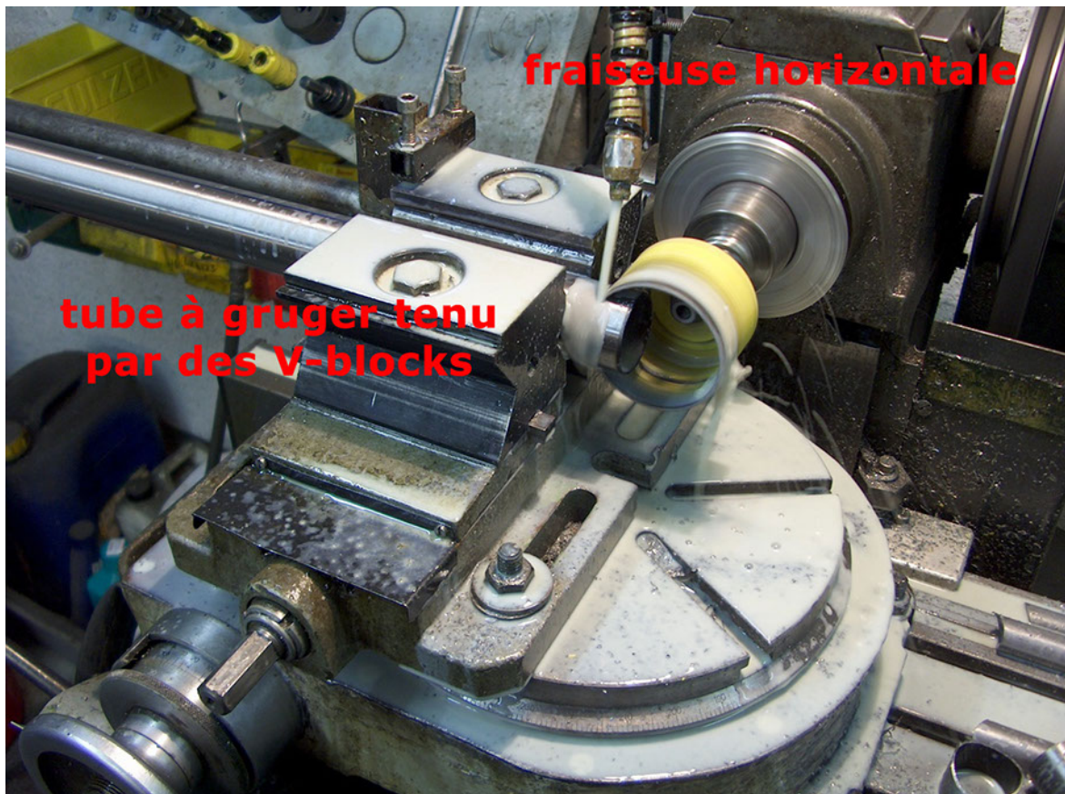
grugeage_sur_fraiseuse_horizontale.jpg
